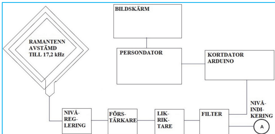
Morsedekoder - Blockschema
